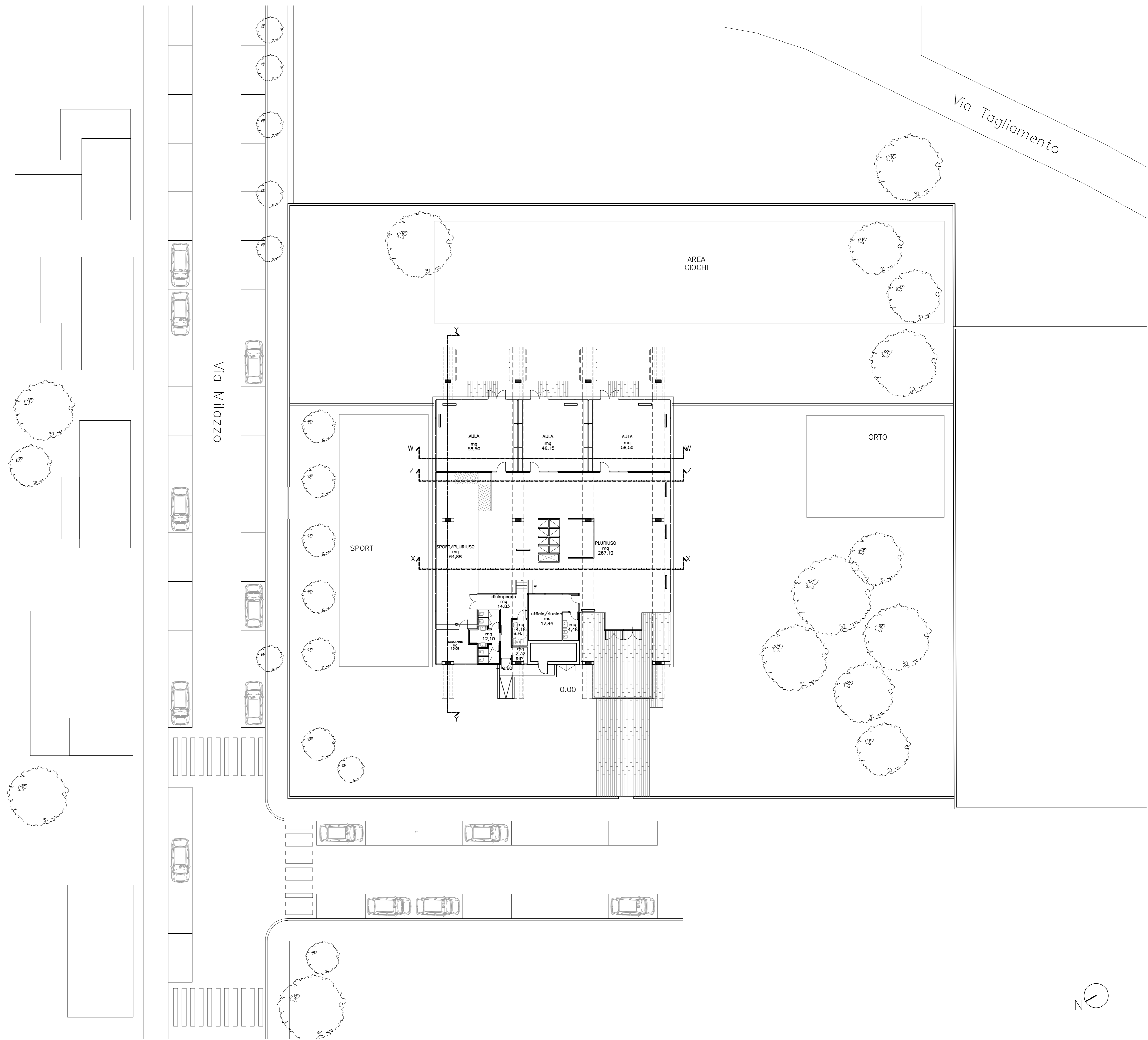
PLANIMETRIA GENERALE POST OPERAM sc. 1:200
