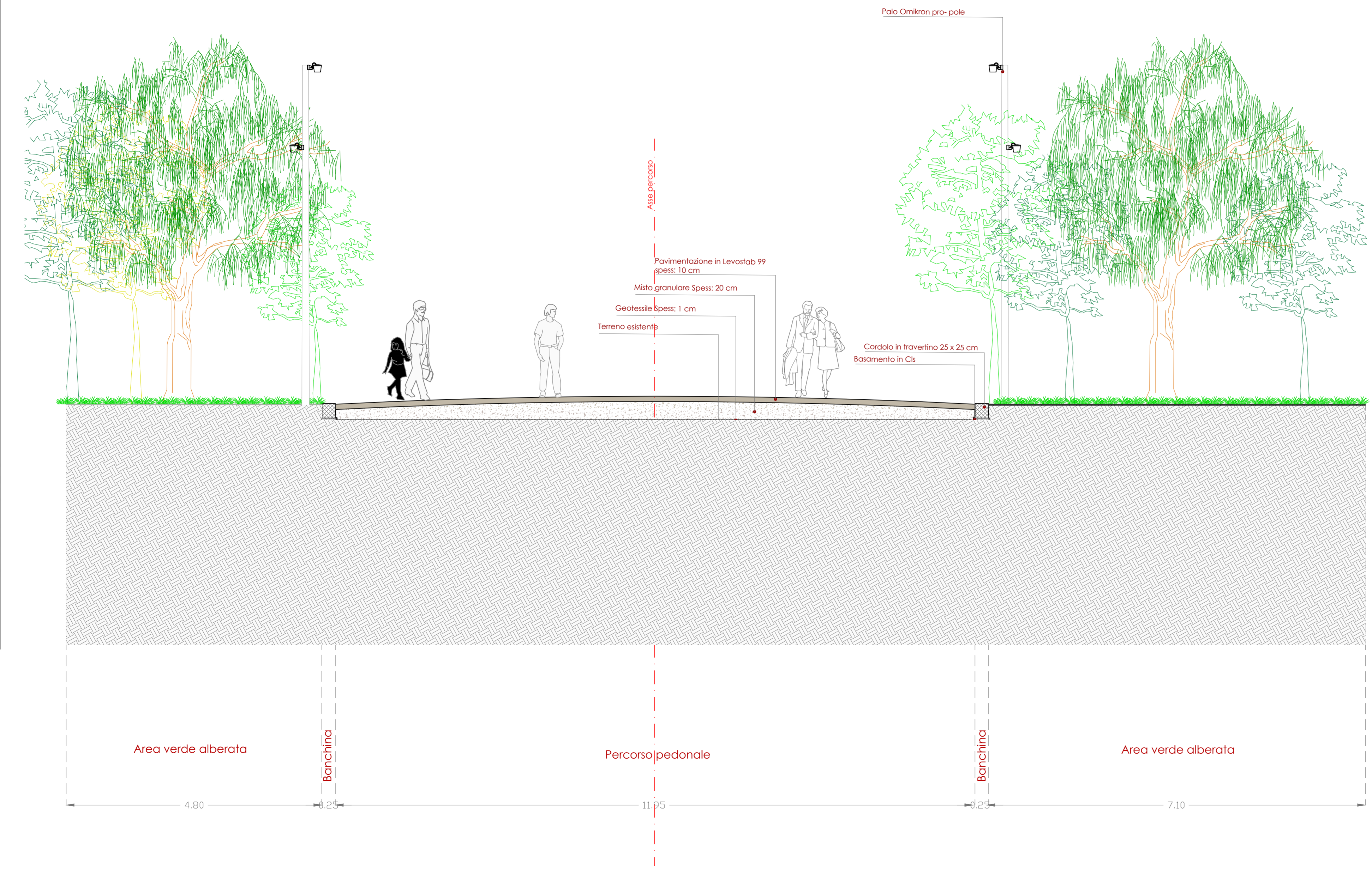
Sezione A Scala 1:50
