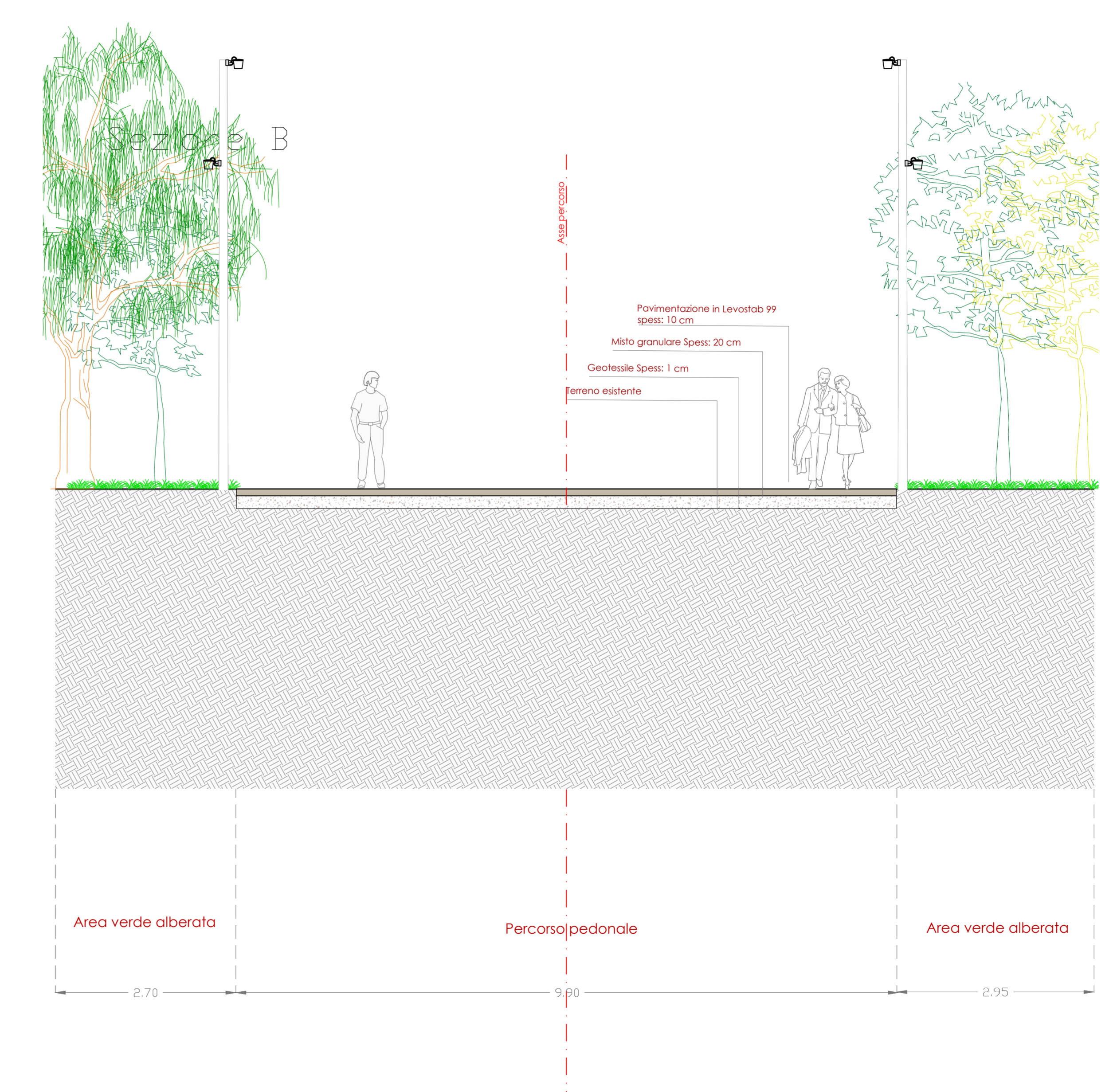
Sezione B Scala 1:50
