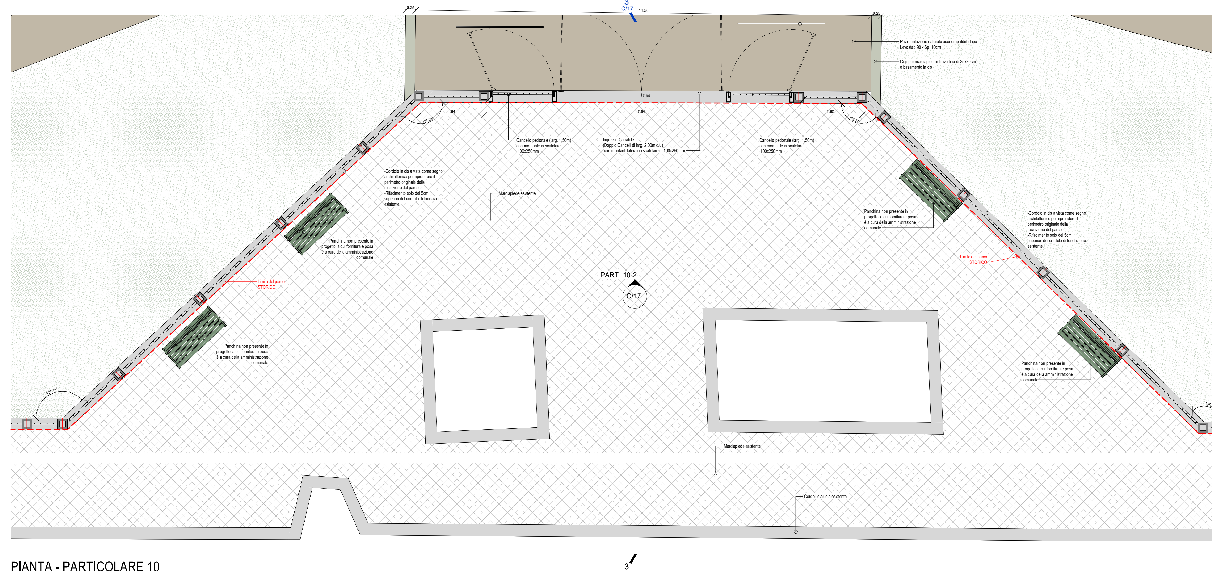
PIANTA - PARTICOLARE 10 Scala 1 : 50
