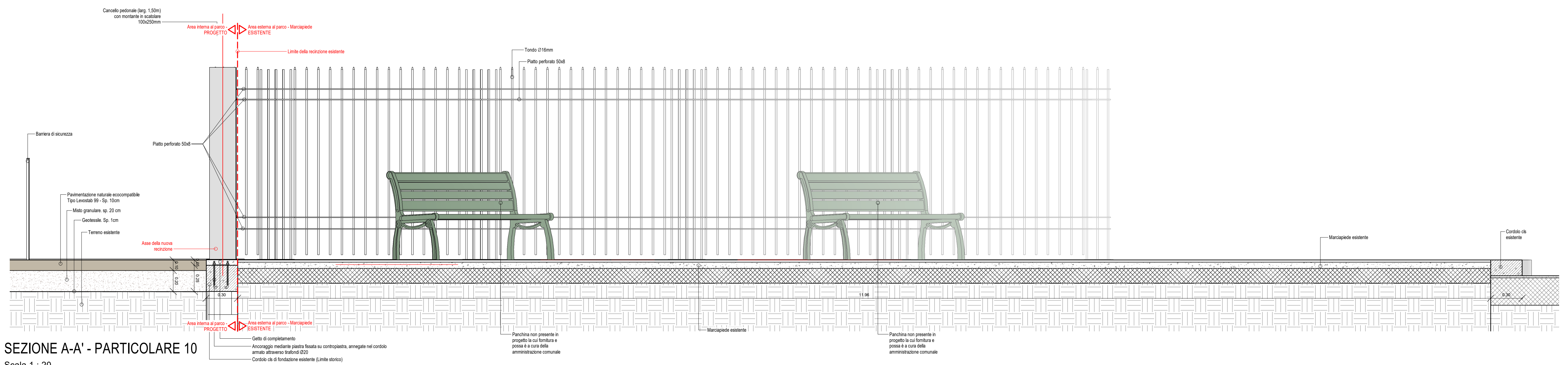
PART. 10 Scala 1 : 50
