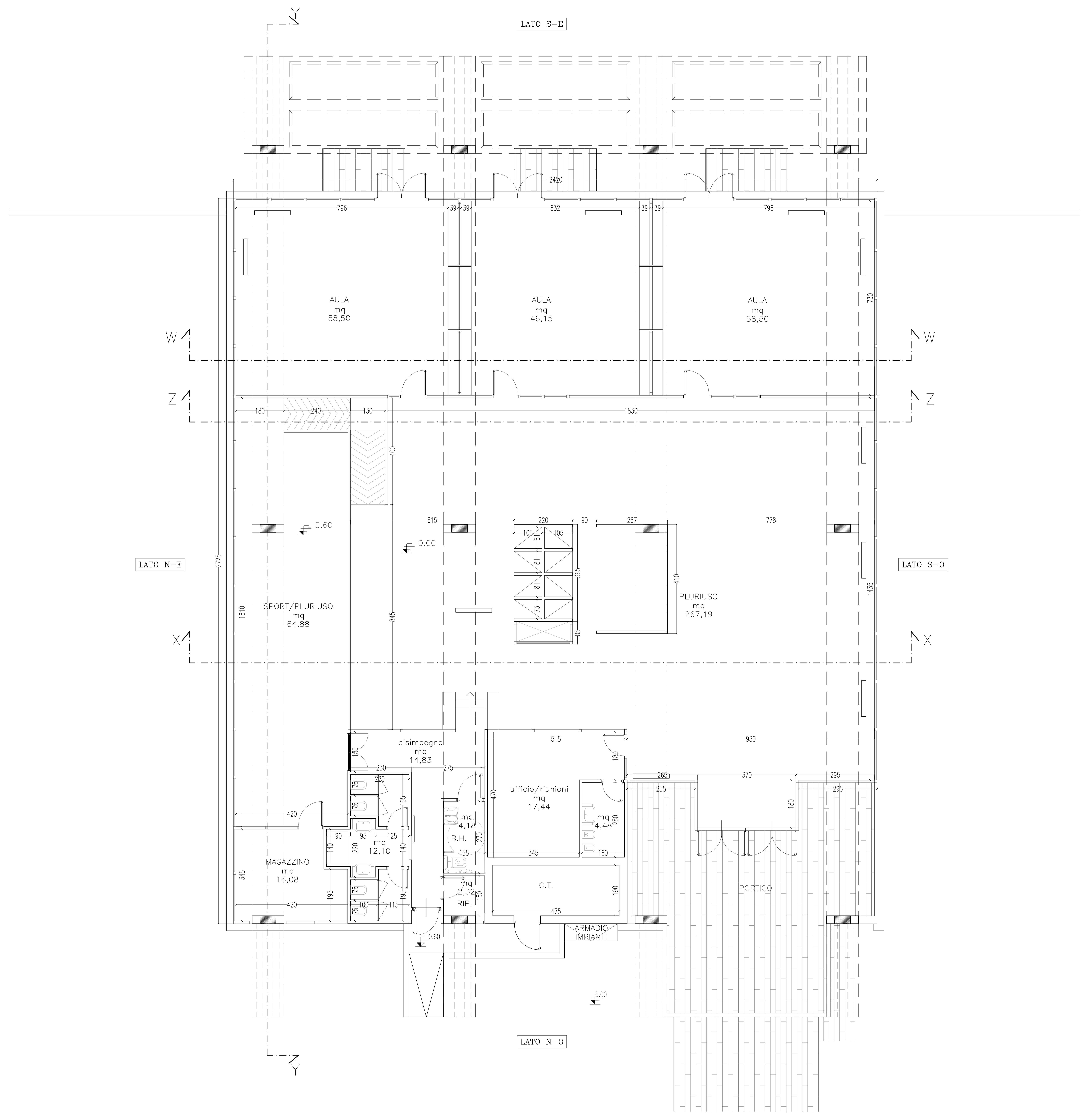
PIANTA PIANO TERRA POST OPERAM sc. 1:50
